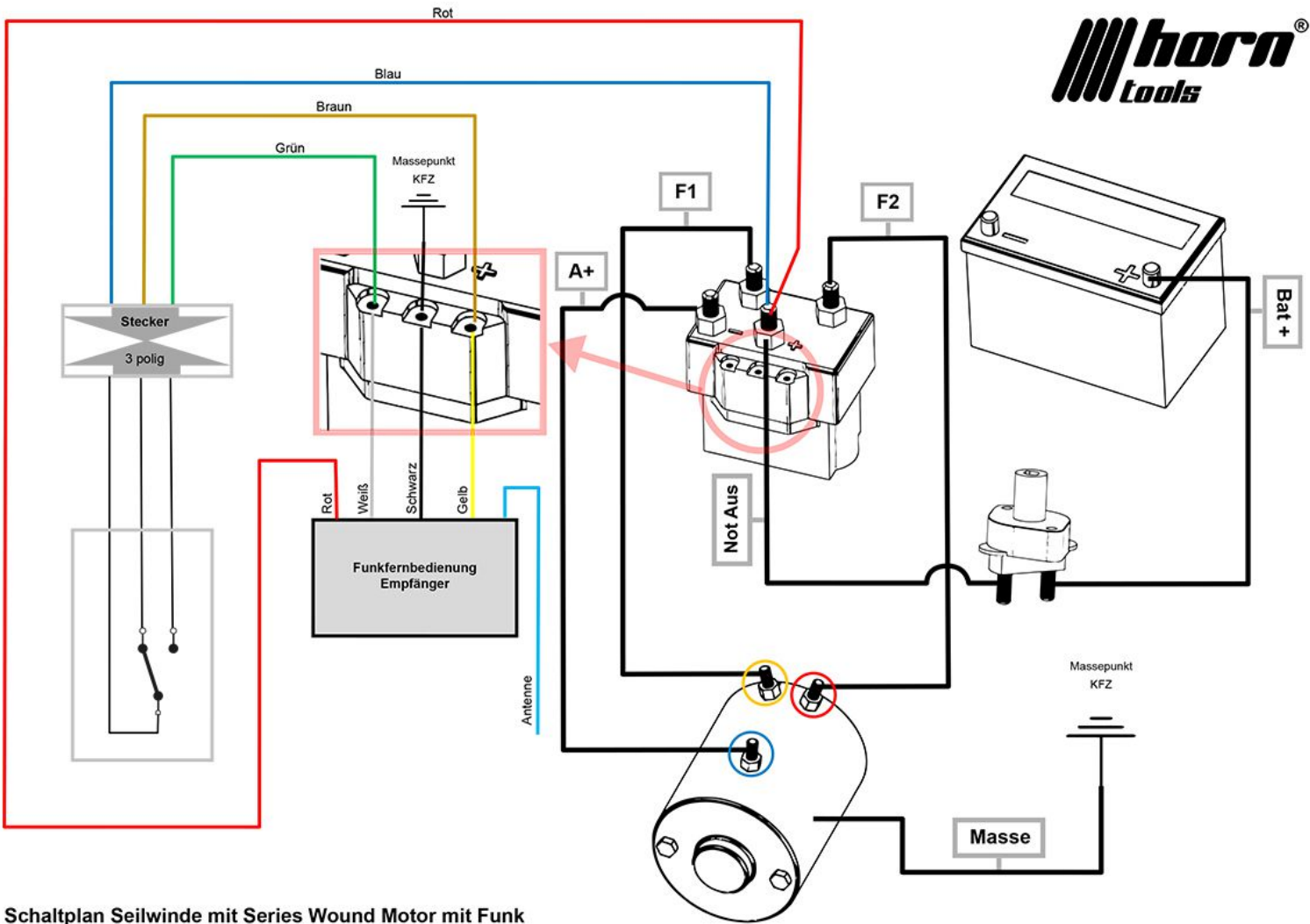
Schaltplan Seilwinde mit Series Wound Motor mit Funk
