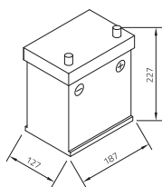
Maße
